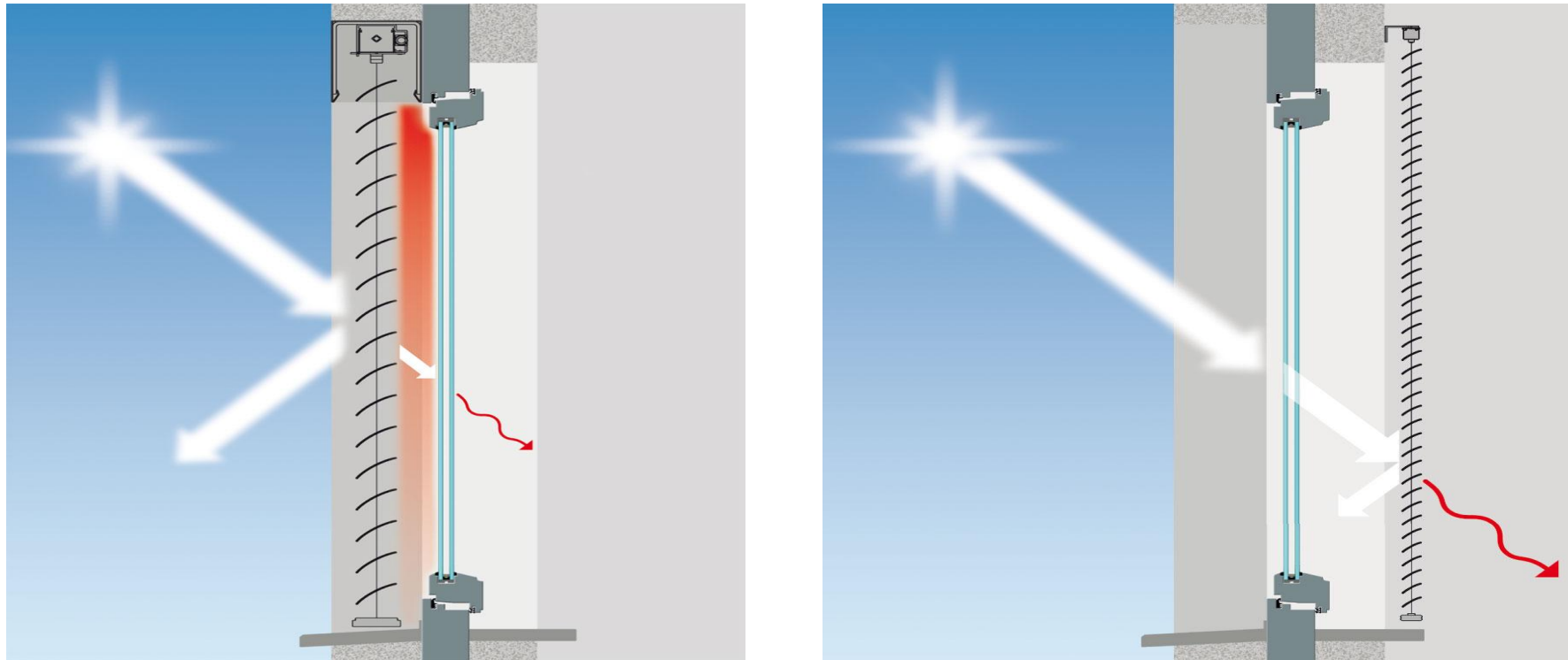
Reduzierung der Aufheizung von Gebäuden durch Außen- und Innensonnenschutz
